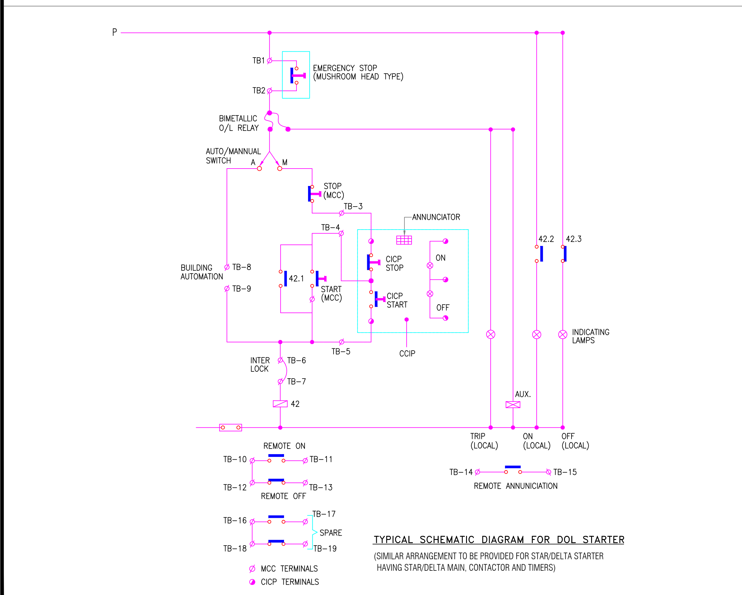
EXHAUST FAN
